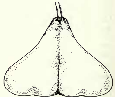
Tyto alba
